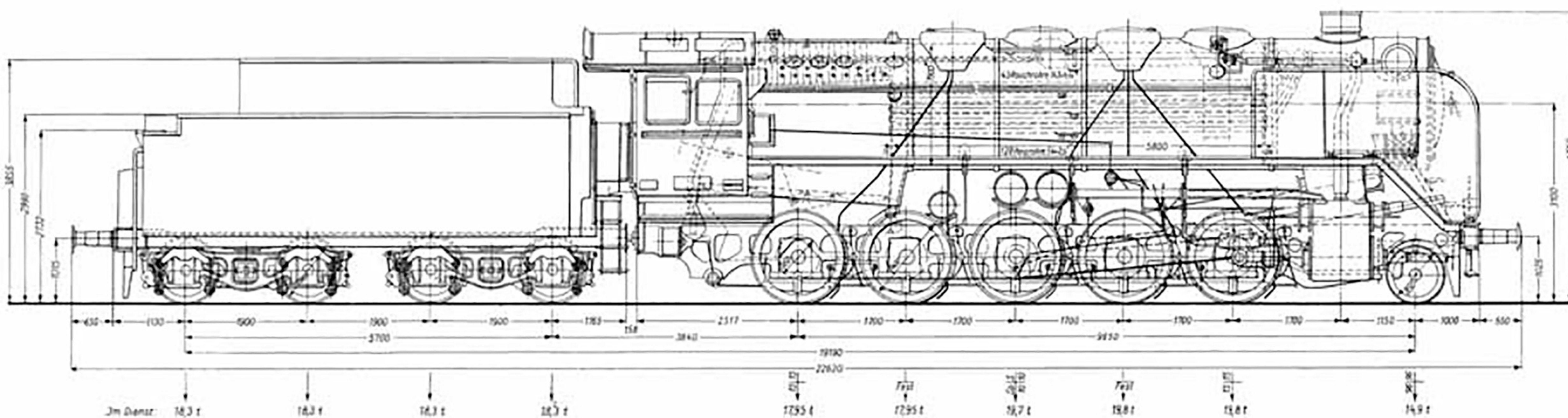
Bild 9. 1' E h 3 Güterzuglokomotive, Baureihe 44, Tender 2' 2' T 34
